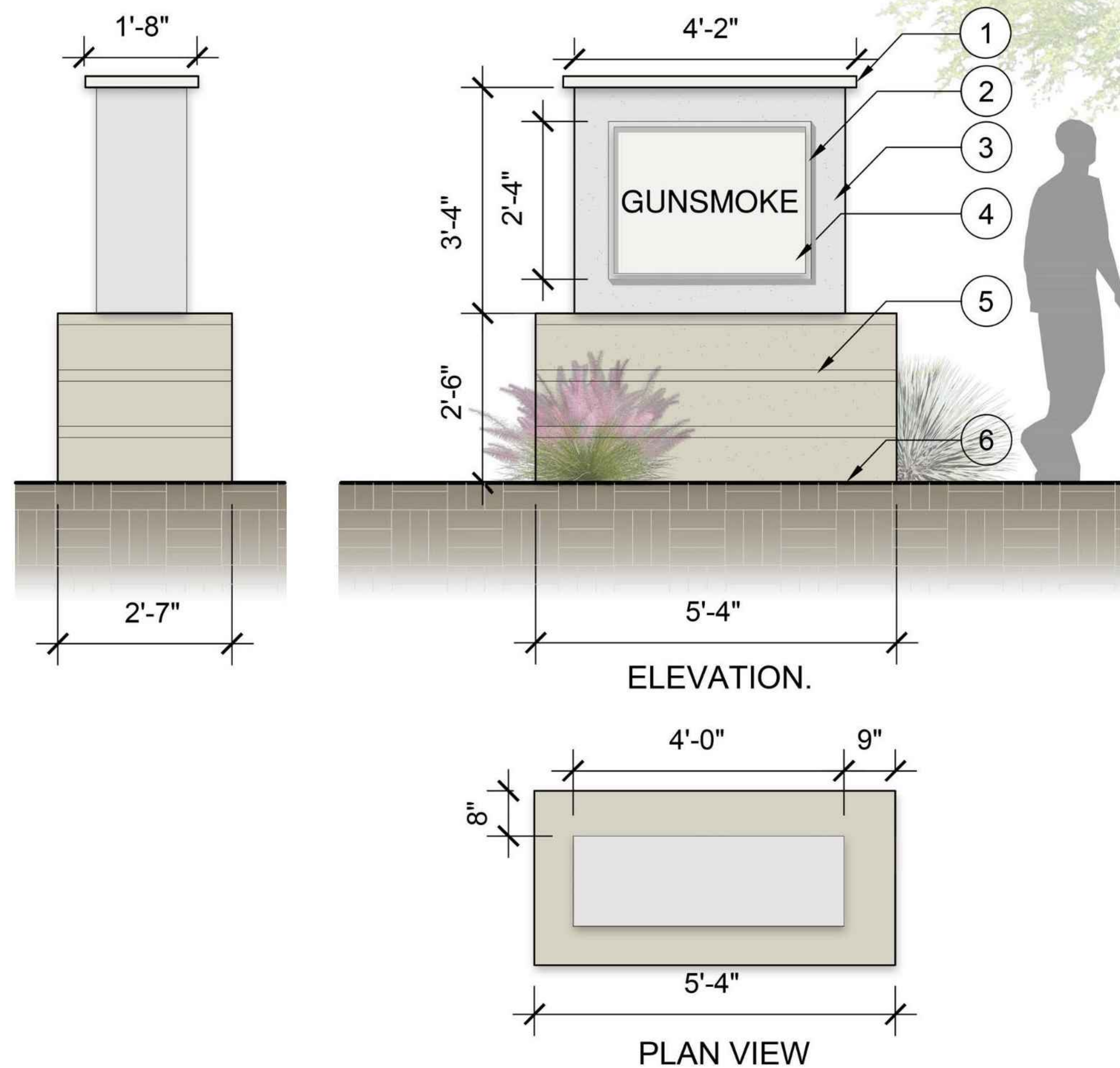
01 SITE MAP MONUMENT
