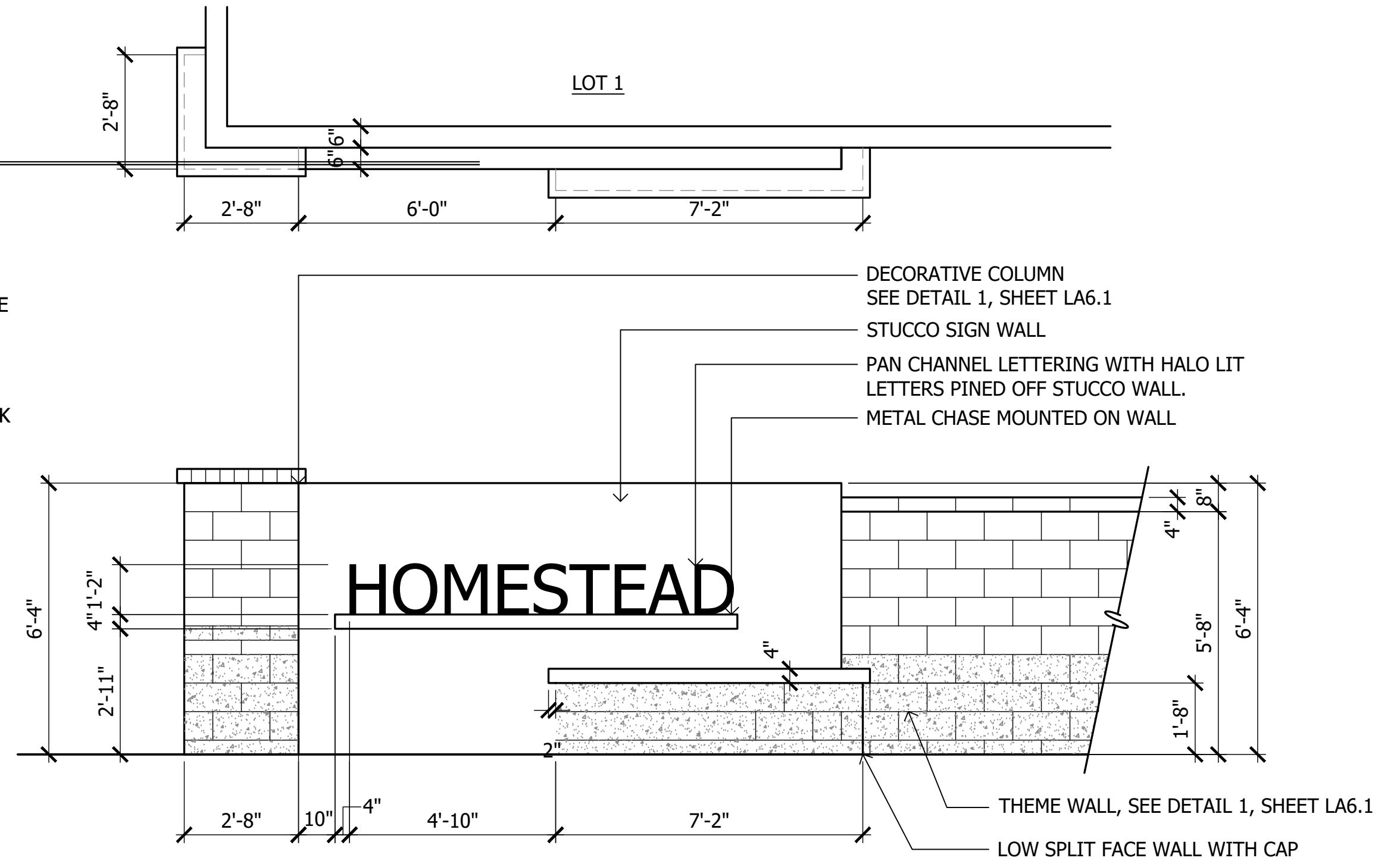
2 Parcel Entry Feature SCALE: 3/8"=1'-0"
